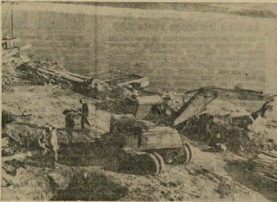
Sneg je zavrl dela za novi most čez Savo v Krškem, vendar gradnje niso ustavili. Z mehanizacijo, s katero je gradbišče dobro opremljeno, si bodo pomagali vse dotlej, dokler ne bo zemlja zmrzovala. Posnetek prikazuje dela na desnem bregu Save, kjer pripravljajo Pionirjevi delavci temelje za novi most (Foto: Ivan Zoran)
