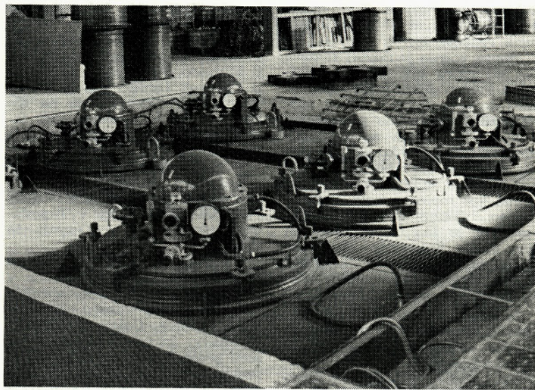
Žarilne peči
