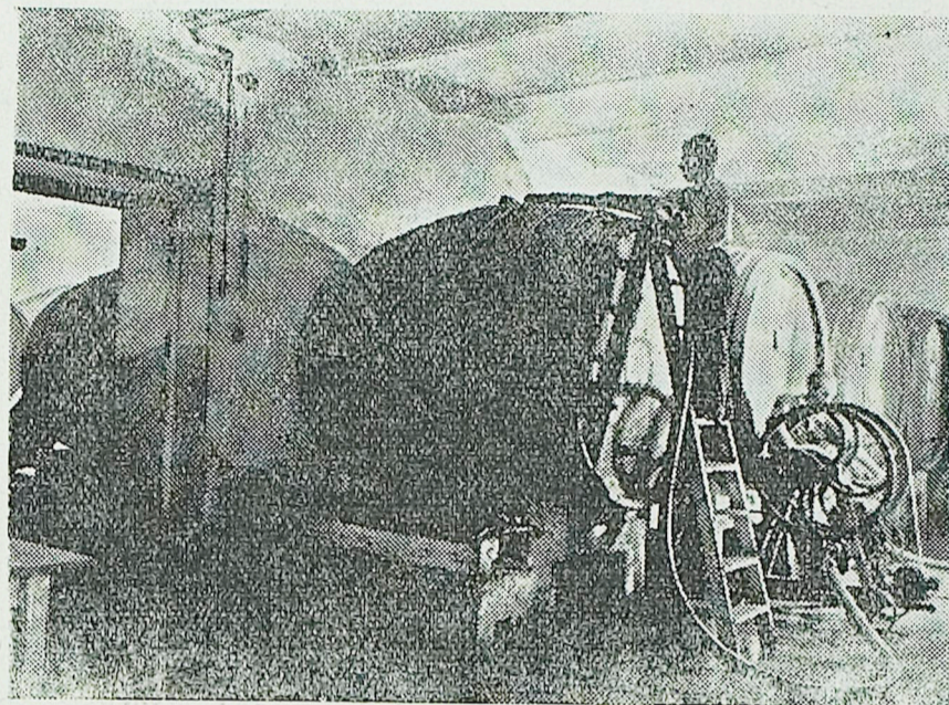
Klet vinarske zadruge v Vipavi, ki ima kapaciteto 60 vagonov vina. Ker je klet za sedanje potrebe že premajhna, imajo v načrtu povečanje kleti, da bo lahko sprejela 100 vagonov vina. Zaradi visoke talne vode je klet zgrajena nad zemljo. — Na sliki vidimo delavce pri pretakanju vina
