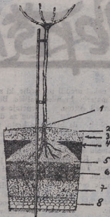
1.) Cepljeno mesto; 2.) Površje zemlje; 3.) Navadna zemlja; 4.) Dobro zrel gnoj pomešan z umetnim gnojili; 5.) Fina zemlja ali preseki; 6.) Zemlja pomešana z zrelem gnojem; 7.) Navadna zemlja; 8.) Drenaža.
