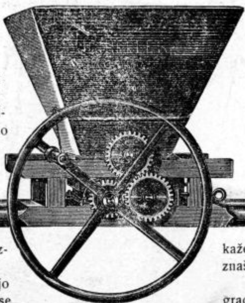
Pod. 50. Grozdna drozgalnica z mešalom.
