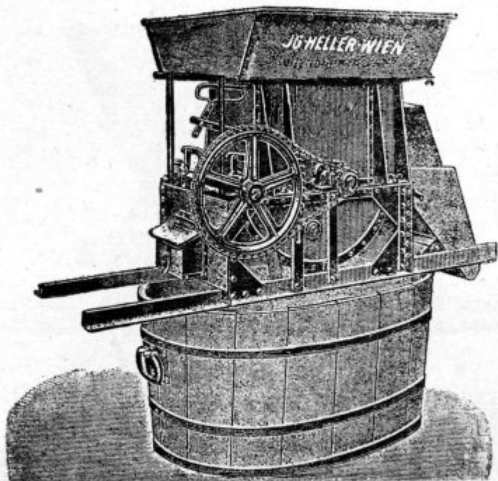
Pod. 51. Centrifugalna drozgalnica za parno moč.
