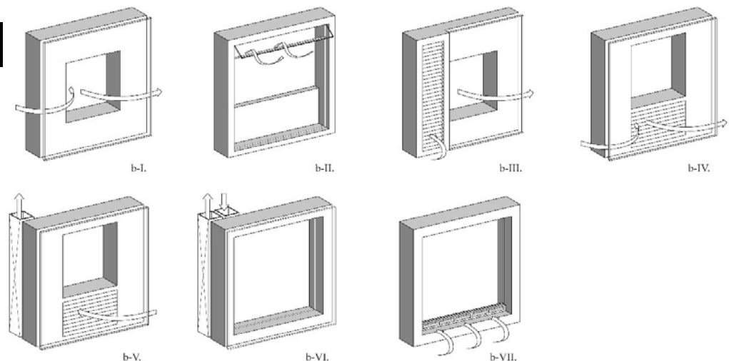
Slika 4: Avtonomni in pol-avtonomni načini prezračevanja (skupina b; I.-VII.).
