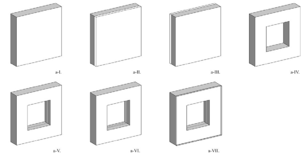
Slika 3: Sheme osnovnih elementov fasad (skupina a; I.-VII.).
