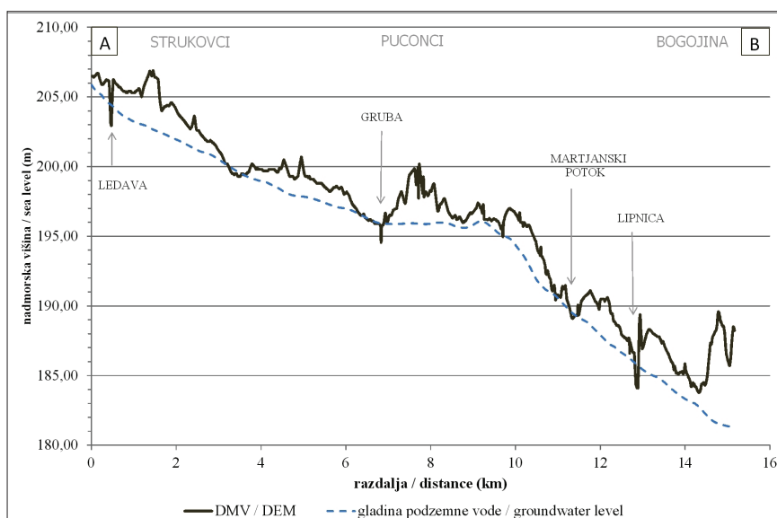
Sl. 3. Interpretiran hidrogeološki profil A – B na Prekmurskem polju (glej sl. 2). Fig. 3. Hydrogeological profile A – B in Prekmursko polje (see Fig. 2).
