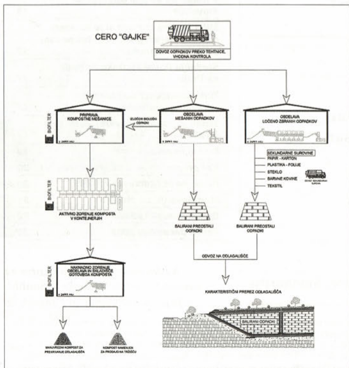
Shematski prikaz pretoka odpadkov na CERO Gajke (avtor sheme: Danijel Prevolšek)
