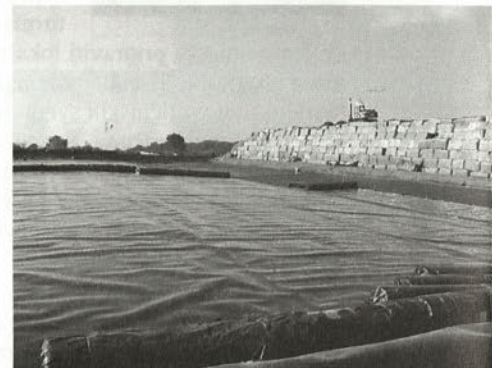
Zaključna faza izgradnje drugega odlagalnega polja. V ozadju prekrivanje zapolnjenega prvega odlagalnega polja.
