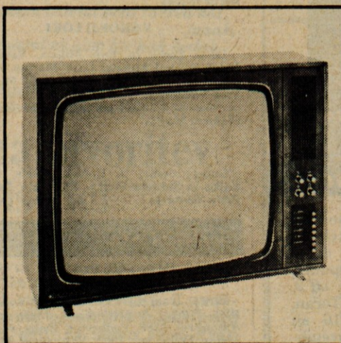
Črno-beli televizor Iskra PANORAMA ARIES: tiskano vezje, 10 elektronk, 7 tranzistorjev, 21 diod, VHF in UHF kanalnik, ekran 61 cm
