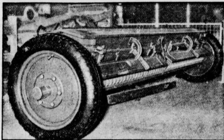
Poljedelski stroj na gumijastih kolesih. Na sedanji kmetijski razstavi v Berlinu so razstavili tudi tale stroji za gnojenje. Stroj teče na gumijastih kolesih, s čimer je delo na polju zelo olajšano.
