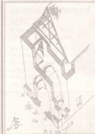
Aksonometrija vzhodnega dela ladje s slavolokom in zvonikom; risal V. Kopač.
