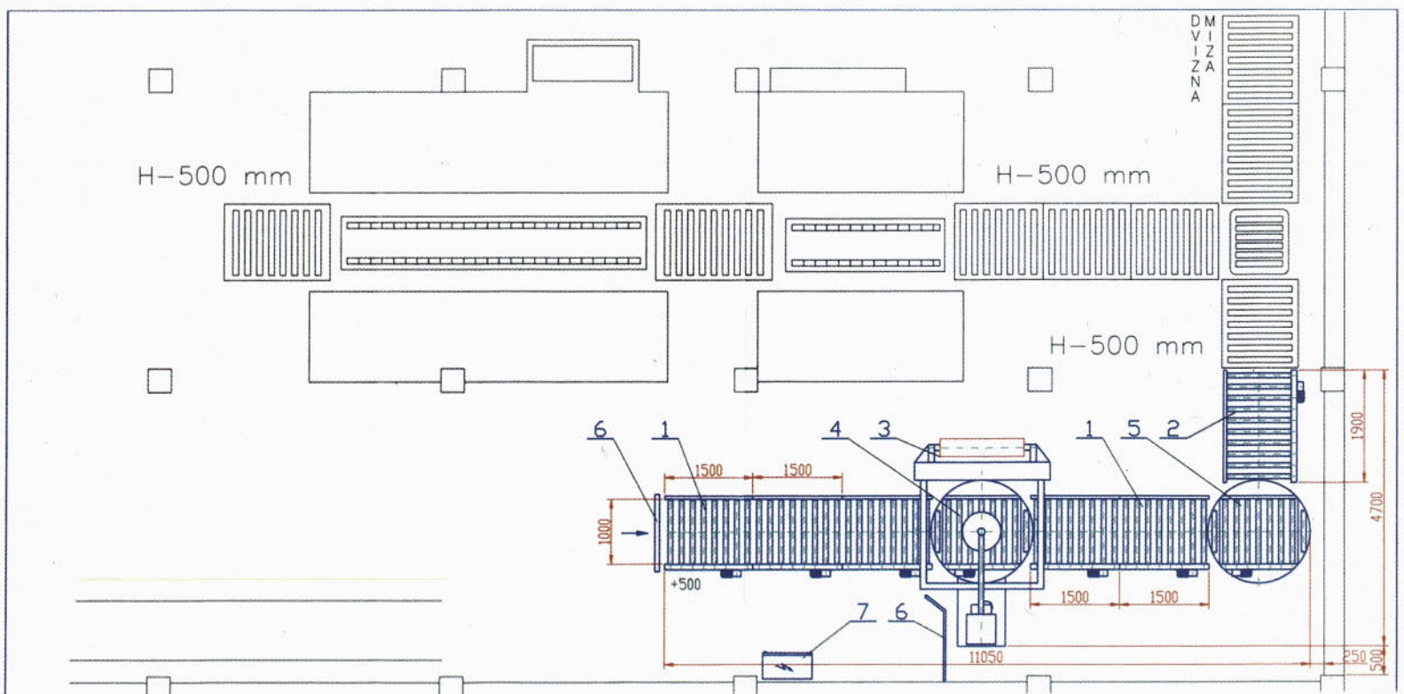
Načrt postavitve stroja za ovijanje palet.
