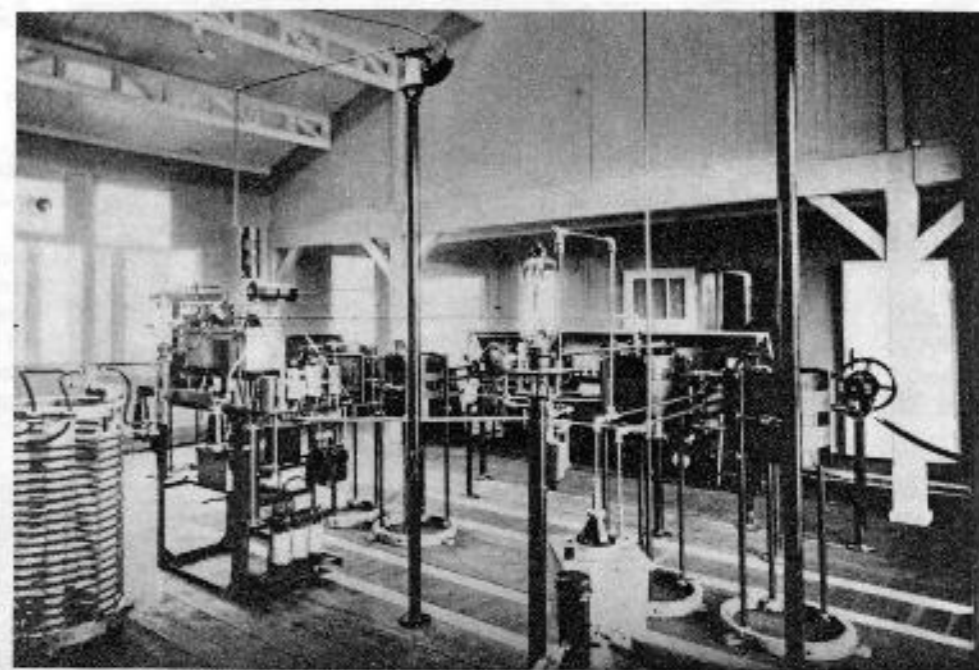
Oddajna aparatura naše radijske postaje v Domžalah. Iz studija v Ljubljani pride sem glas po telefonu, ti aparati ga pa izpremeje v radijske valove, ki jih pošilja potem antena v svet.
