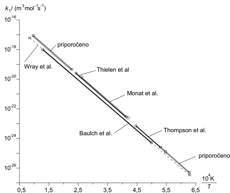
Sl. 1. Odvisnost k_1 = k(1/T) za reakcijo O + N_2 \rightarrow NO + N [13]
