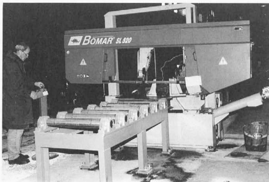
Tračna žaga v adjustazi kovačnice
