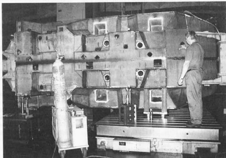
V STO v kratkem pričakujejo naročilo še 16 valukov – na fotografiji je varjenje školjke valuka.
