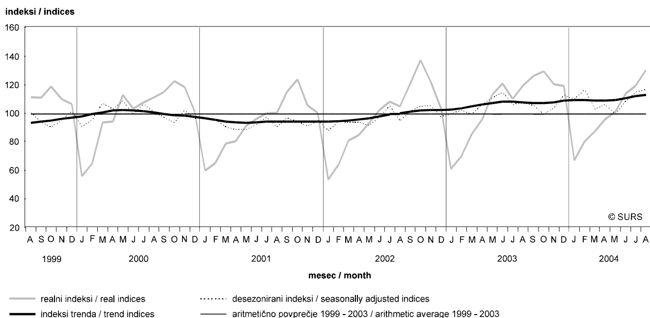
Slika 1: Indeksi vrednosti opravljenih gradbenih del, Slovenija, avgust 1999 - avgust 2004
