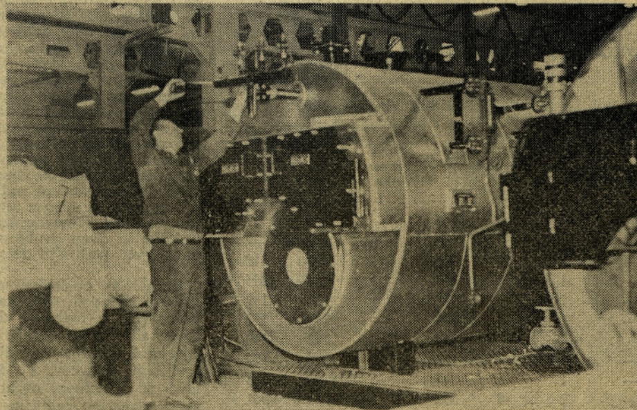
Zahtevna montaža kotlov za ogrevanje stanovanjskih objektov
