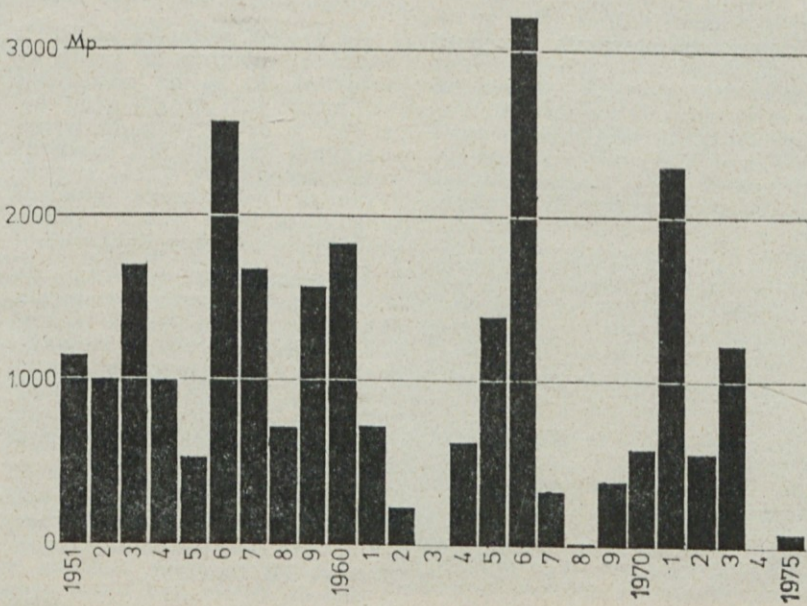
Naročila turbinske opreme za domače hidroelektrarne v LITOSTROJU po dobavnih rokih v letih 1951 do 1975
