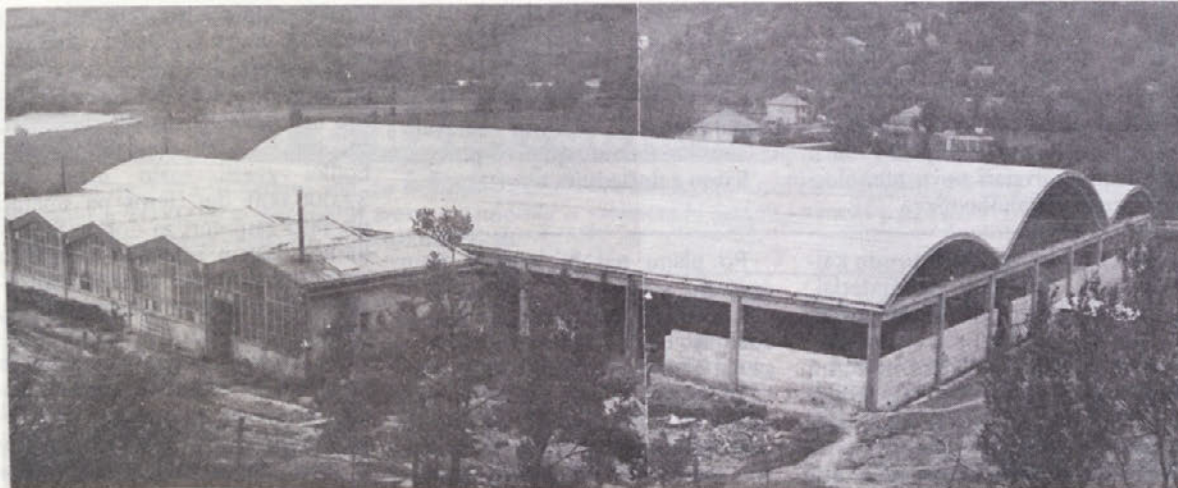
TOGREL proizvodna dvorana za BEBITRIKO v Kulen Vakufu. V ospredju v levem delu slike so dosedanji tovarniški prostori, ki bi jih s streho vred brez težav spravili v polovico ene izmed treh novih TOGREL vzporednic
