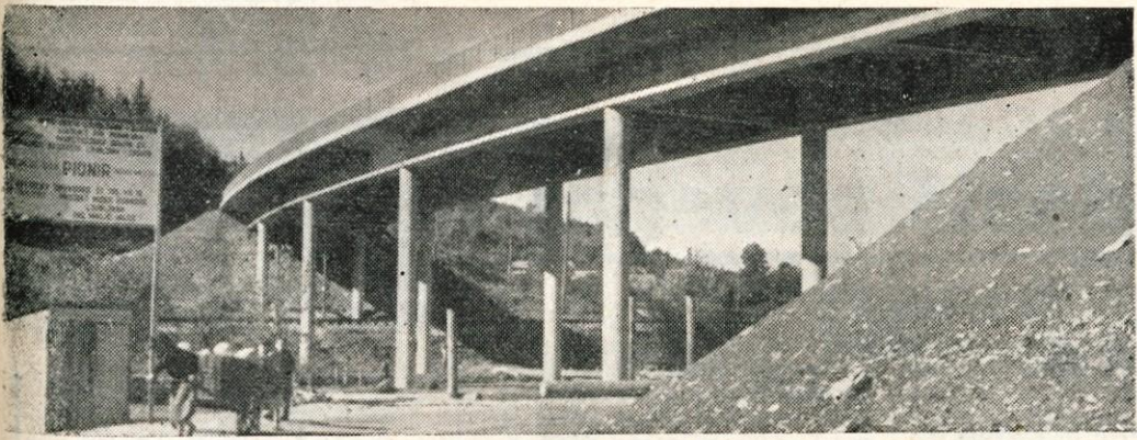
V soboto popoldne so zaključili asfaltiranje avtomobilske ceste od Ljubljane do Zagreba. Zgrajenega je že 79 km asfaltne in betonskega vozišča. Vse tako kaže, da bo cesta dograjena prej, kot je bilo prvotno določeno. Mladinske delovne brigade morajo zdaj opraviti še nekaj manjših del, glavna svečanost pa bo 23. novembra. — Na sliki levo vidite mogočen nadvoz nove avtomobilske ceste pri Ponikvah
