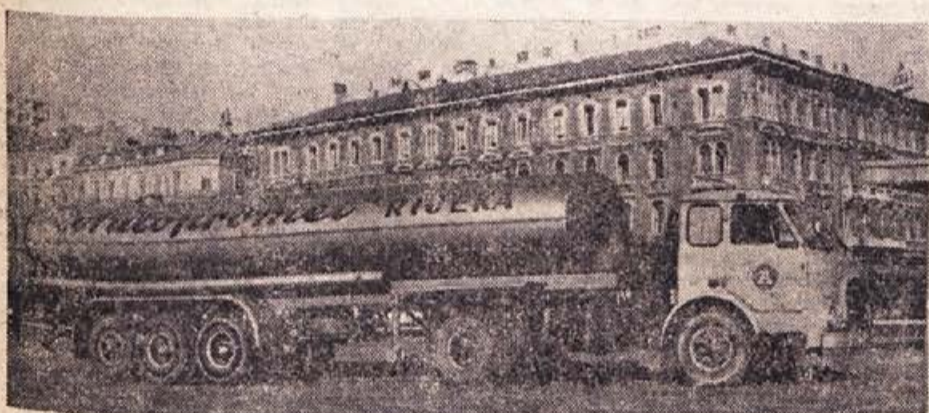
Cisterna za prevoz vina tipa PPV - 26 lahko prepelje 20.000 litrov vina hkrati. »Avto promet Reka« ima dve taki cisterni in sta bili letos že 20-krat na Poljskem. Obe cisterni je izdelalo kočevsko podjetje »Itas« oktobra lani
