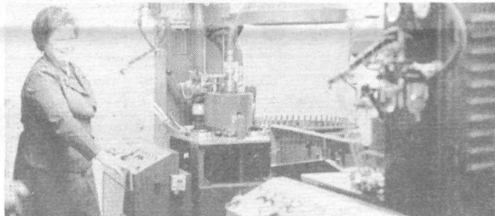
Nad 40 milijonov vredna popolnoma sinhronizirana linija SACMI za izdelavo navojnih zapork 28 krat 15 mm bo nekaj mesecev kovala te zelo iskane zaporke v začasni prostorih stare delavnice za izdelavo aluminijastih zapork. Pričakujejo, da bo lahko stekla na stalnem mestu v veliki proizvodni dvorani proti koncu letošnjega leta.
