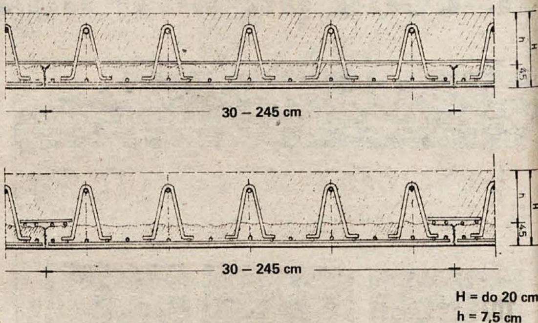
PREREZI OPAŽNIH BETONSKIH ELEMENTOV
