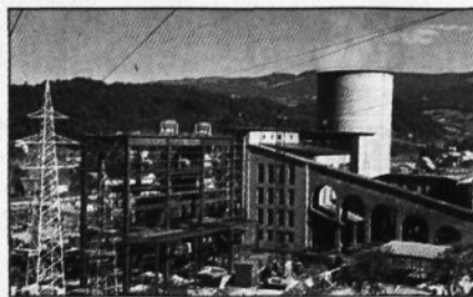
Izgradnja nosilne konstrukcije kotlov WB in dimnikov v letu 1974
