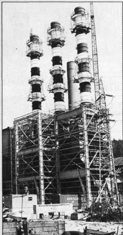
Glavni pogonski objekt - pripravljen za zapiranje kotlovnice (1974) Dimnike je po kosih sestavljajal 90 metrov visok žerjav.
