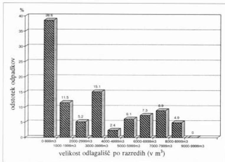
Deleži odpadkov po velikostnih razredih neurejenih odlagališč
