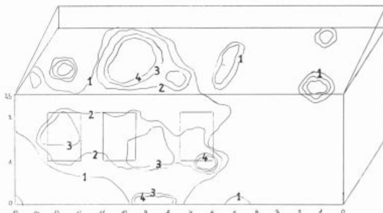
Slika 7: Izodoze na pročelju in strehi zgradbe
