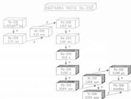
Slika 2: Torijeva razpadna vrsta
