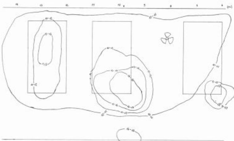
Slika 8: Izodoze na pročelju in na zazidanih oknih
