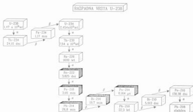
Slika 1: Uranova razpadna vrsta
