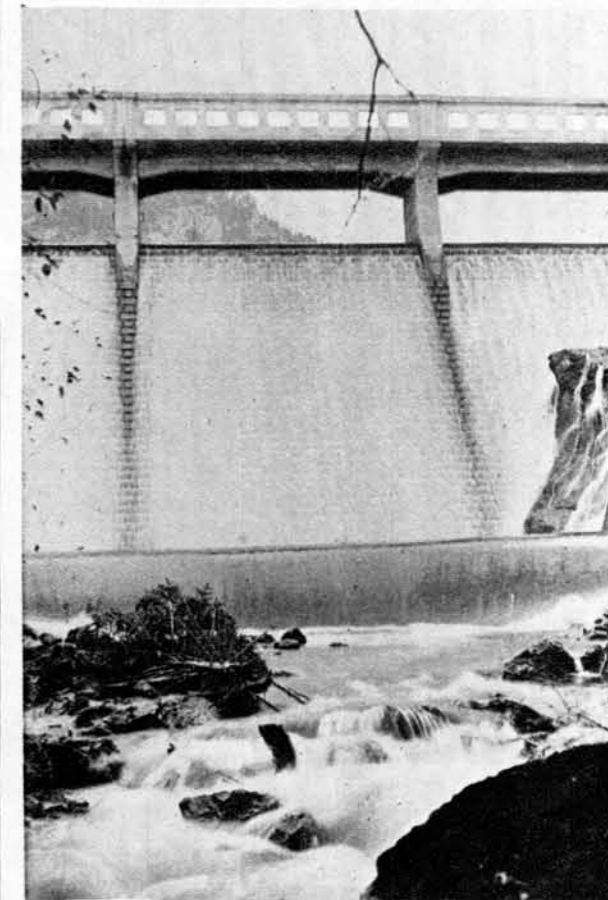
Jez deželne elektrarne na Završnici.
