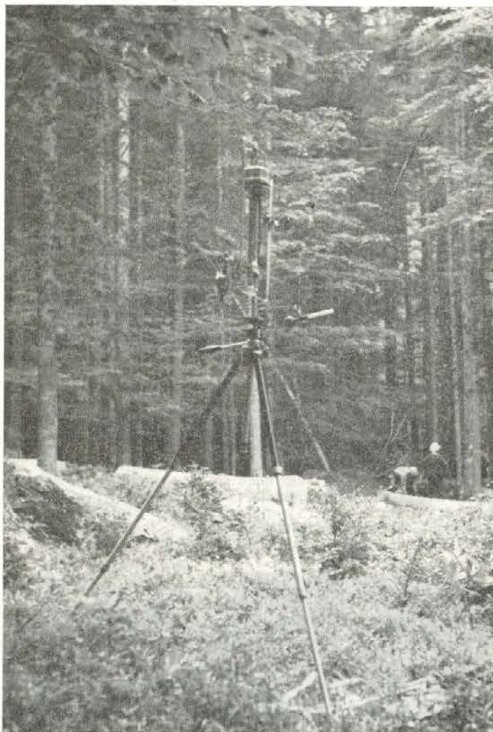
S to aparaturo se meri temperatura zraka, relativna vlaga in brzina gibanja zraka (prepih, veter). Iz podatkov je mogoče oceniti klimatske pogoje. — Foto: Janko Sušnik
