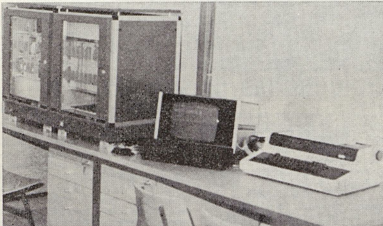
Del računalniške opreme: zbirna postaja, centralna računalniška enota (levo), monitor (v sredini), tastatura in printer
