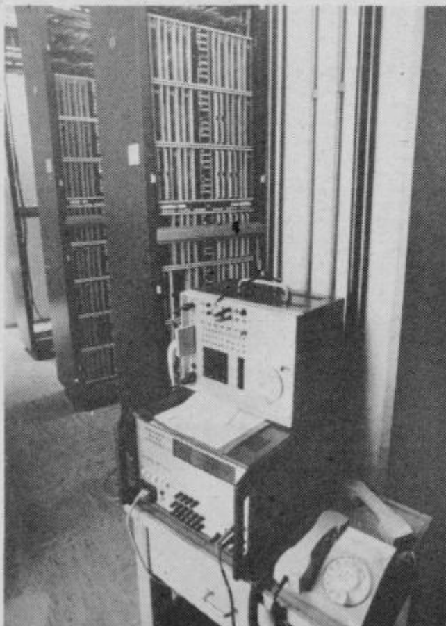
Da bi v novi centrali delalo vse tako kot je treba, so potrebne tudi naprave za nadzor in merjenje.
