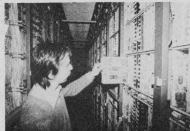
Novo centralo na Golovcu sestavlja približno 14.000 takih enot elektronskih vezij, ki jih kaže Bojan Gorjanc.
