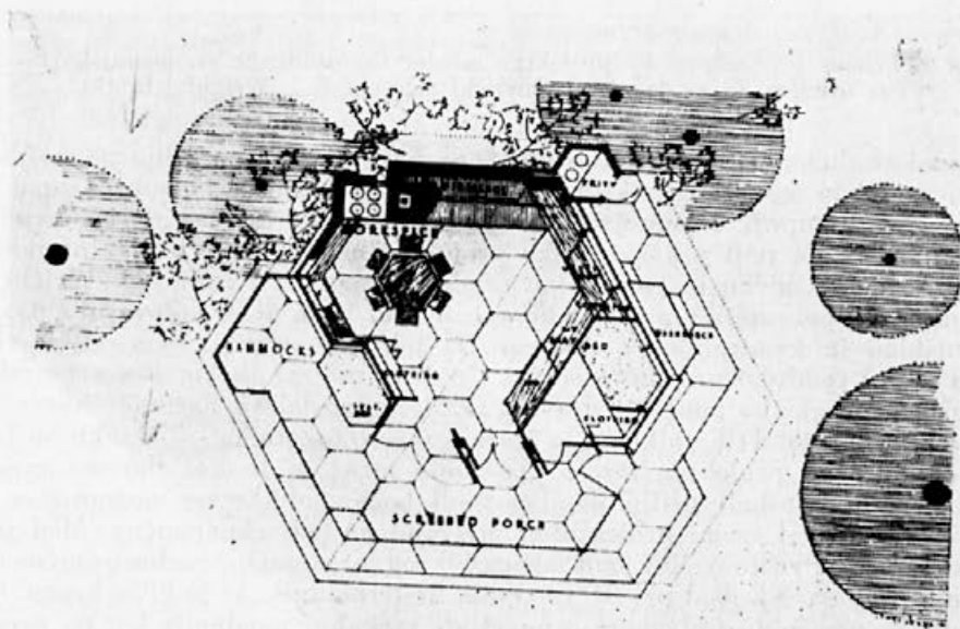
Slika 1. Primer šesterokotniške projektne mreže ameriškega arhitekta F. L. Wrighta: Tloris hiše za gosta na Leigh Stevens Ranch Group pri Yemassee, South Carolina. Hiša je bila zgrajena leta 1940.
