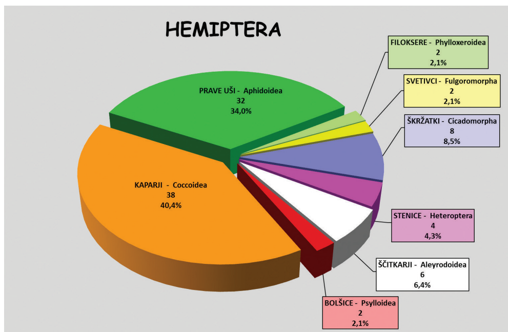
Sl. 2: Struktura tujerodnih rastlinojedih žuželk iz reda Hemiptera v Sloveniji.
