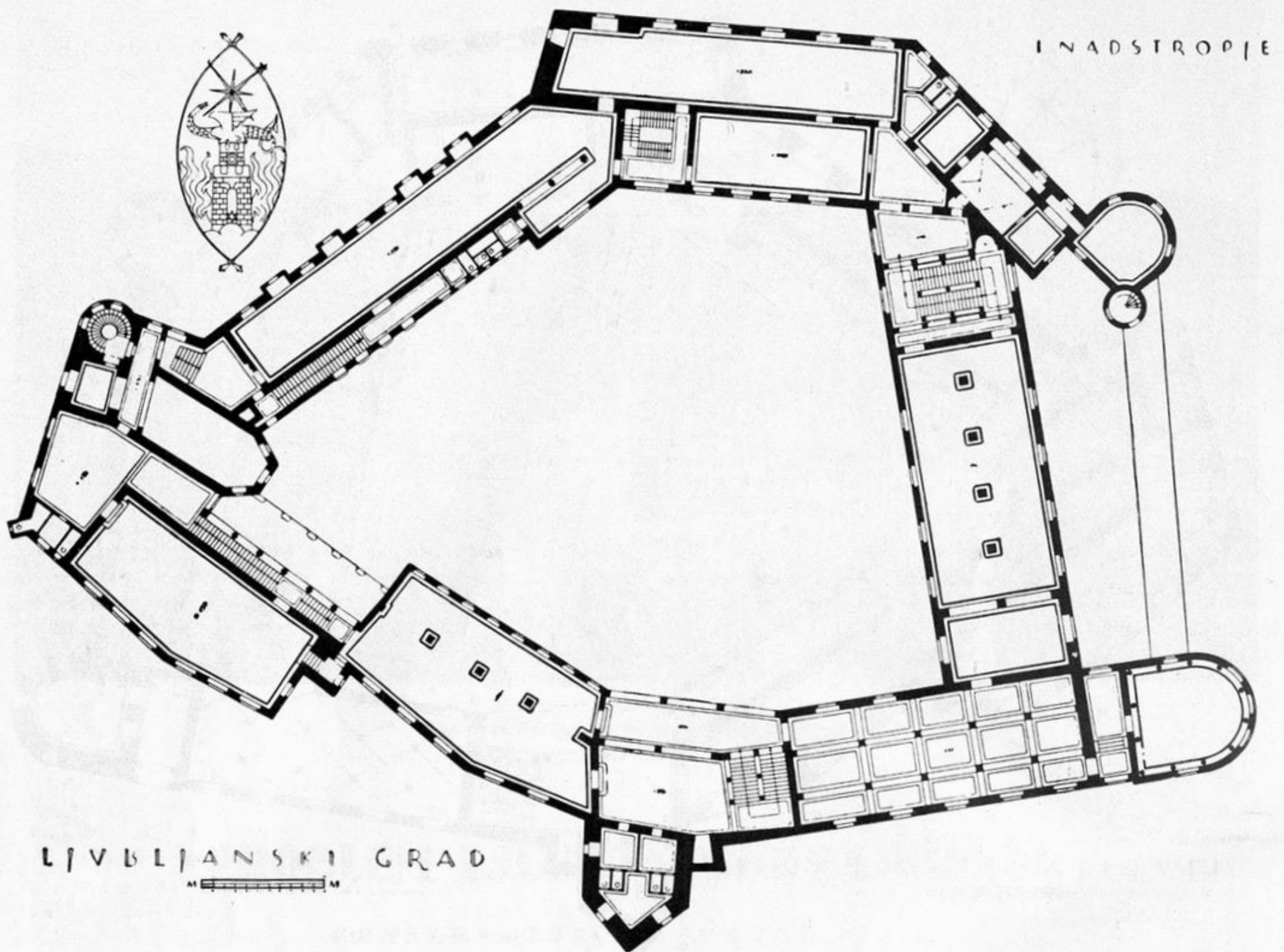
Plečnikov projekt za preureditev ljubljanskega gradu
