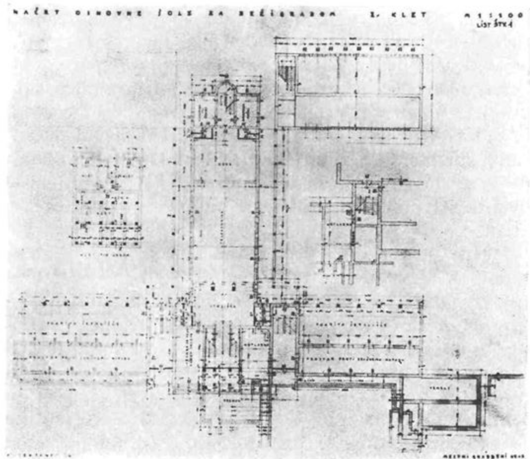
Tloris prve kletne etaže
