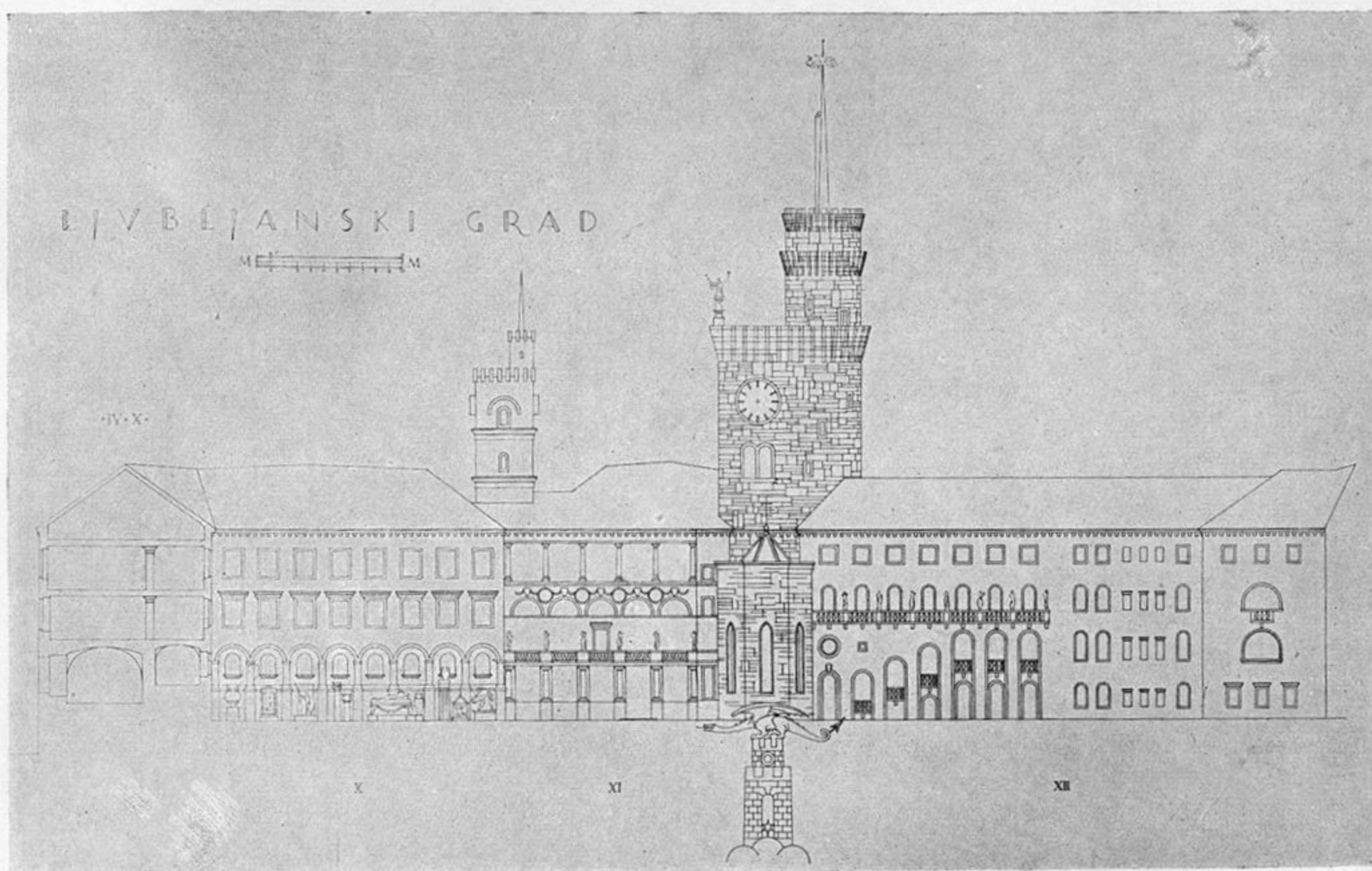
Razvija jugozapadna, zapadna in severna fasada dvorišča ljubljanskega gradu po Plečnikovem projektu. (K članku: Problem ljubljanskega gradu)
