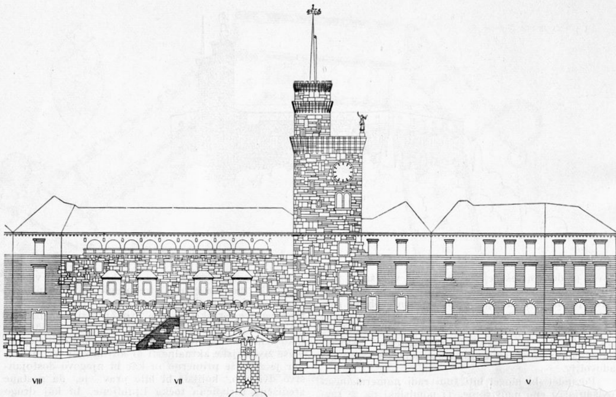
Razvita zapadna in jugozapadna fasada ljubljanskega gradu po Plečnikovem projektu. (K članku : Problem ljubljanskega gradu)
