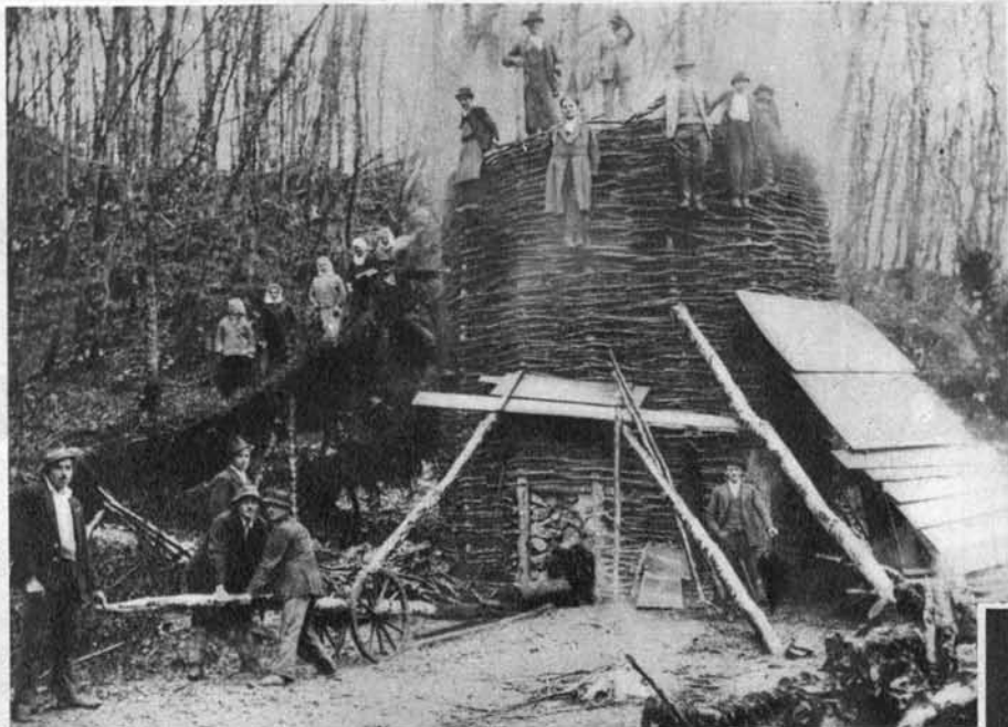
Primitivna apnenica, ki jih najdemo pri nas se tu in tam po kmetih (last L. Lundra iz Cerovca pri Trebelnem). Spredaj je dobro videti še tako zvanega skaštrunac, s katerim porivajo v ogenj cele hlode.
