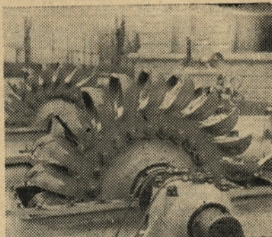
Novo turbine izdelane v Litostroju
