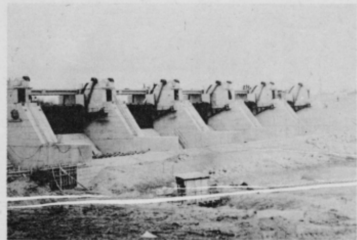
Odtočna stran zapornic pri Markovcih za HC SD 2 Formin. Foto: J. Vrabl
