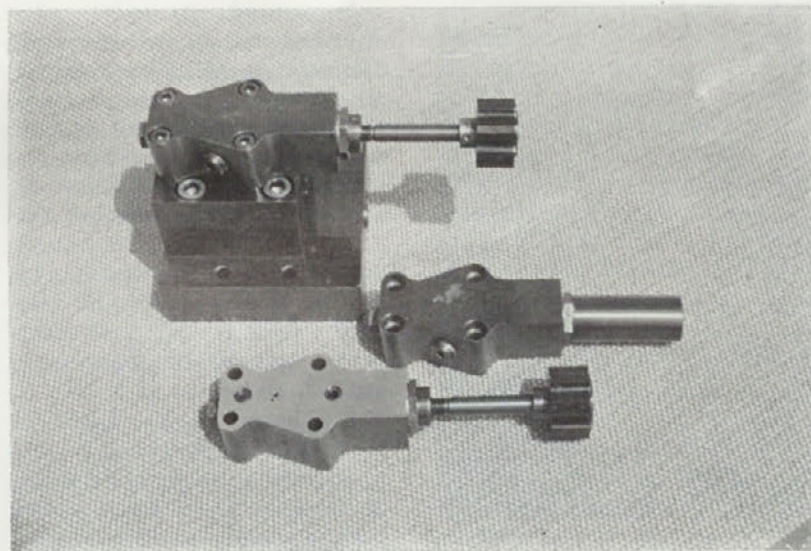
Regulatorji tlaka
