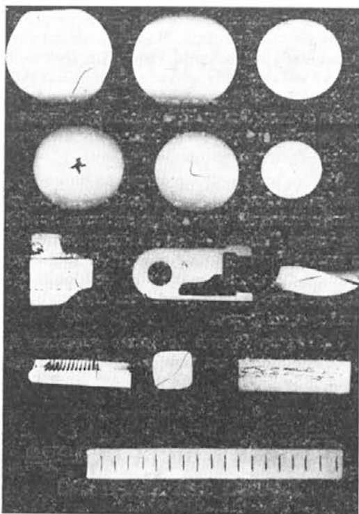
Slika 3: z ultrazvokom najdene napake v jeklu, ki so vidne po razrezovanju in fero-fluksanju. Zgoraj levo proti desni: a) razpoka zaradi hladnega kovanja, b) kosmiči — razpoke zaradi vodika, dolge 30 mm, c) kosmiči — dolžine do 10 mm, d) lunker v kovani palici, e) in f) kovaški križ — razpoke na visoko legiranih jeklih zaradi hladnega kovanja, g) lunker v odlivku, h) razpoka v sredini brzoreznega svedra, i) prečna razpoka na navoju palice za vrtnanje nafte, j) prečna razpoka v gredici, k) podkožne razpoke blizu površine gredice, l) prečne razpoke v vlečni palici, m) razpoka v palici za vrtnanje nafte, nastala po varjenju
