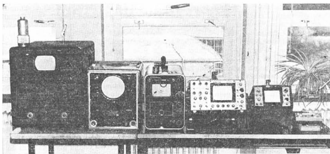
Slika 2: od leve na desno: ultrazvočni aparati iz leta 1952, 1959, 1961, 1970, 1971, 1972. Zgoraj ultrazvočne glave
