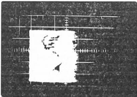
Slika 4 — B slika — z ultrazvokom najdeni defekti v platiranem nožu. Temne lise so defektna mesta. Slika je posneta z vrtečo se ultrazvočno glavo v treh sekundah
