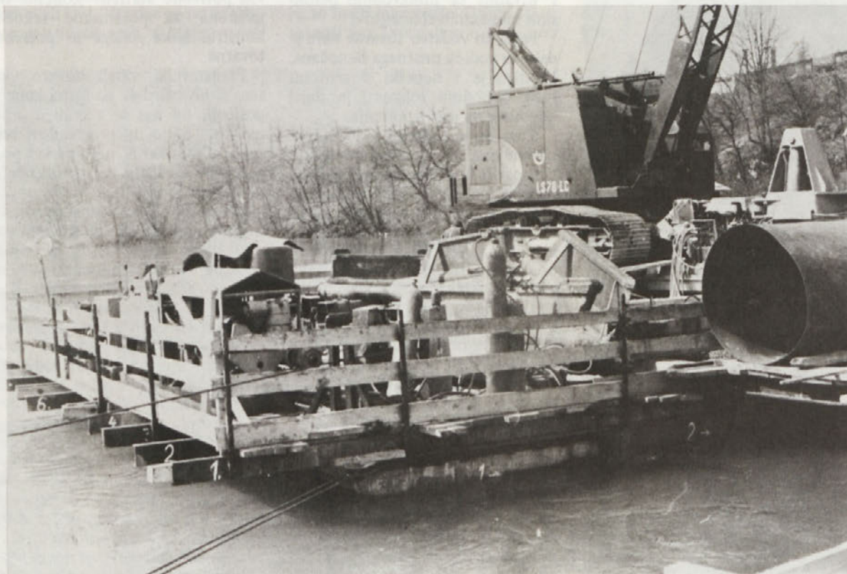
Splav z bagerjem in napravami Geotehnike na gradbišču novega mostu v Novem mestu. V desnem kotu v ospredju slike vidite jekleni Benotto pilot, kakršne zabijajo v rečno dno
