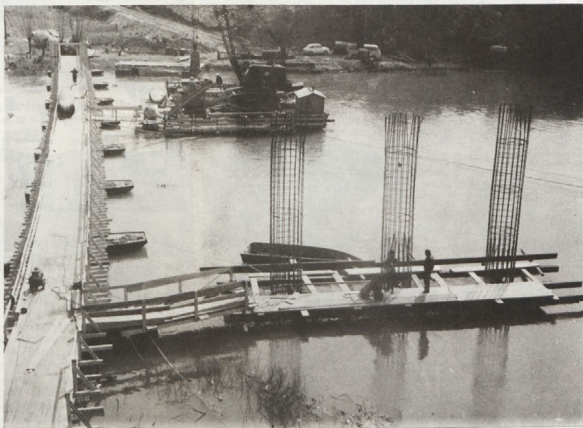
Pogled na pontonski most, prvi niz treh stebrov novega mostu ob levem bregu, za katere so Benotto piloti že zabiti in armatura že štrli visoko iz vode ter splav s stroji in napravami Geotehnike na gradbišču novega mostu v Novem mestu
