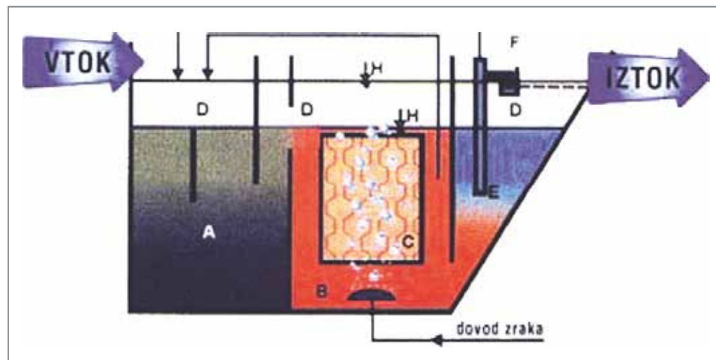
Presek tipične biološke MKČN (A – dotočni prekat, B – čistilni prekat, C – SBR, D – iztok iz ČN)
