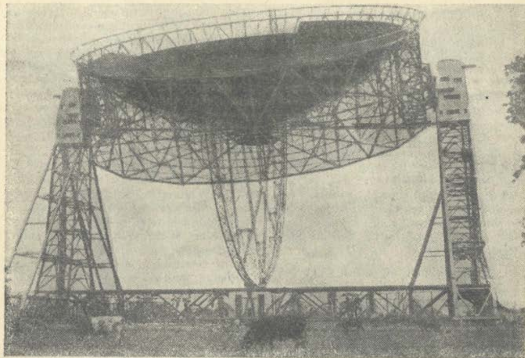
Osemdeset metrov meri v premeru zrcalo radijskega teleskopa vseučilišča v Manchesteru. Zanj so porabili 2000 ton jekla
