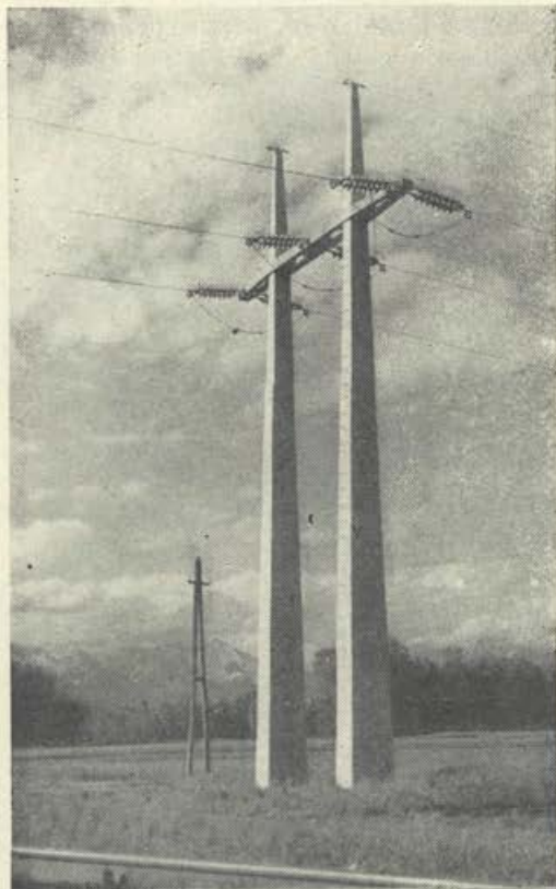
Jambor 110.000-voltnega trofaznega daljnovoda na Sorškem polju pri Medvodah; višina jambora je 17 m, razdalja med žicami 4,5 m
