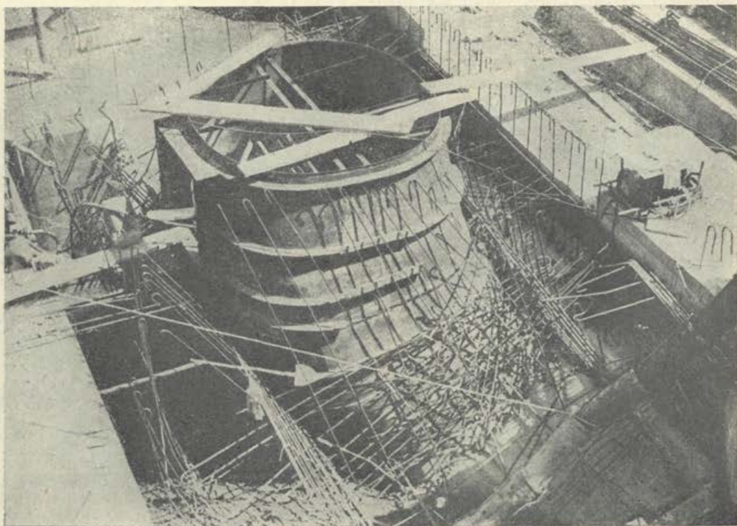
Odtočna cev vodne turbine 12.000 konjskih sil v hidroelektrarni Medvode na Savi med vbetoniranjem
