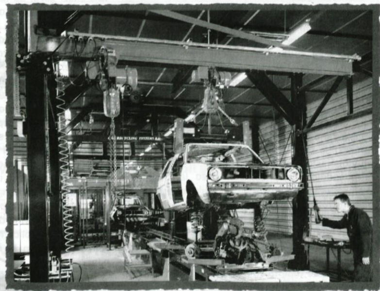
Slike spodaj: Ostali tehnološki procesi v razstavjalnici.
