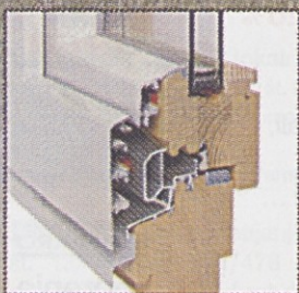
Leseno okno z alu oblogo
