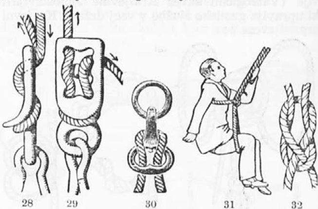
28., 29. in 30. Priprava, ki jo uporablja gasilec za lastno spuščanje po vrvi — 31. in 32. Razine vrste vozlov, ki jih uporabljamo za reševanje
