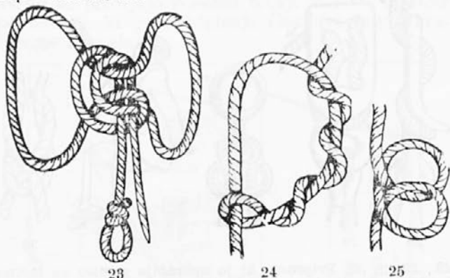
23., 24. in 25. Razne vrste vozlov, ki jih uporabljamo za reševanje
