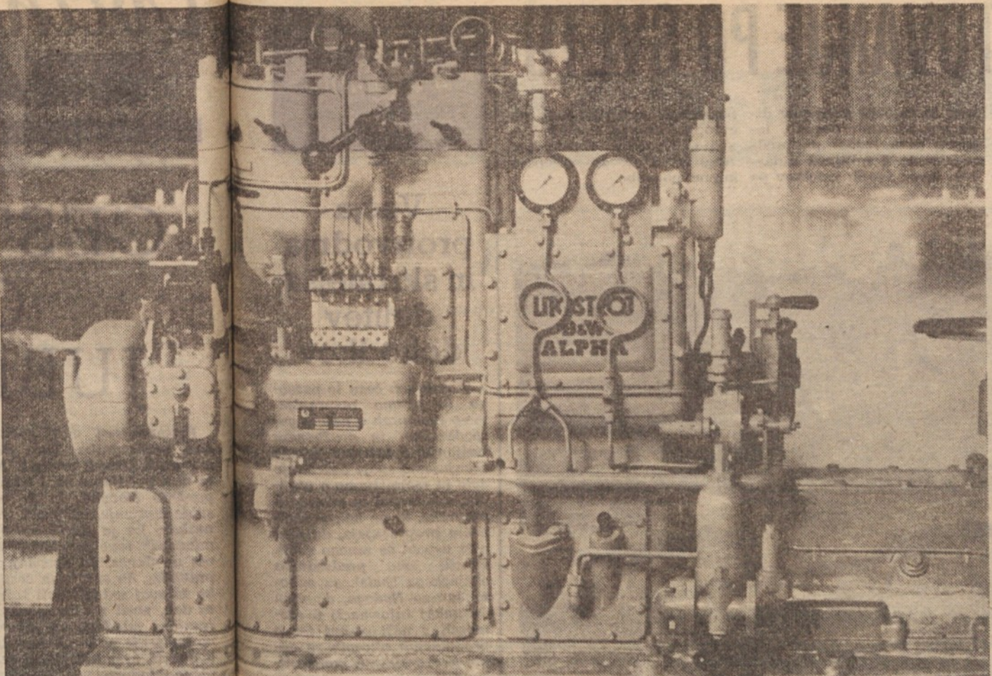
Pomembnih proizvodov Litostroja: dvocilindrski Diesel motorji
