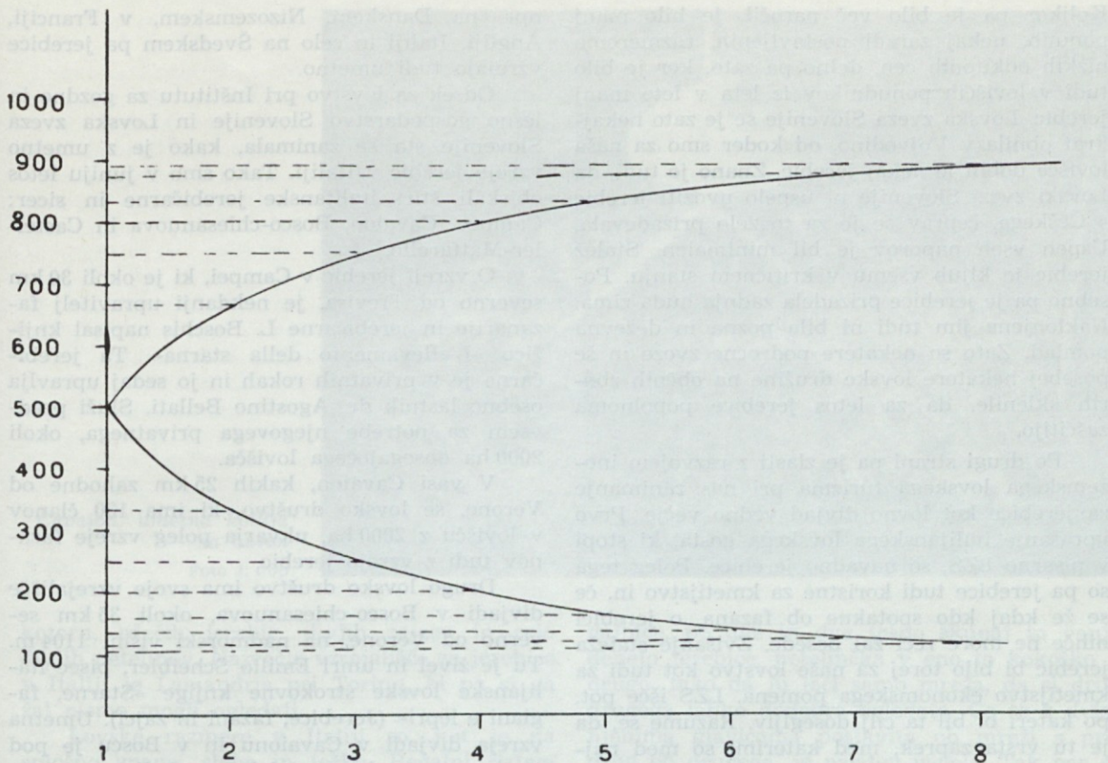
Grafični prikaz medsebojne odvisnosti povprečnega letnega prirastka po enoti, matičnega fonda in skupnega letnega prirastka male zaščitene divjadi
