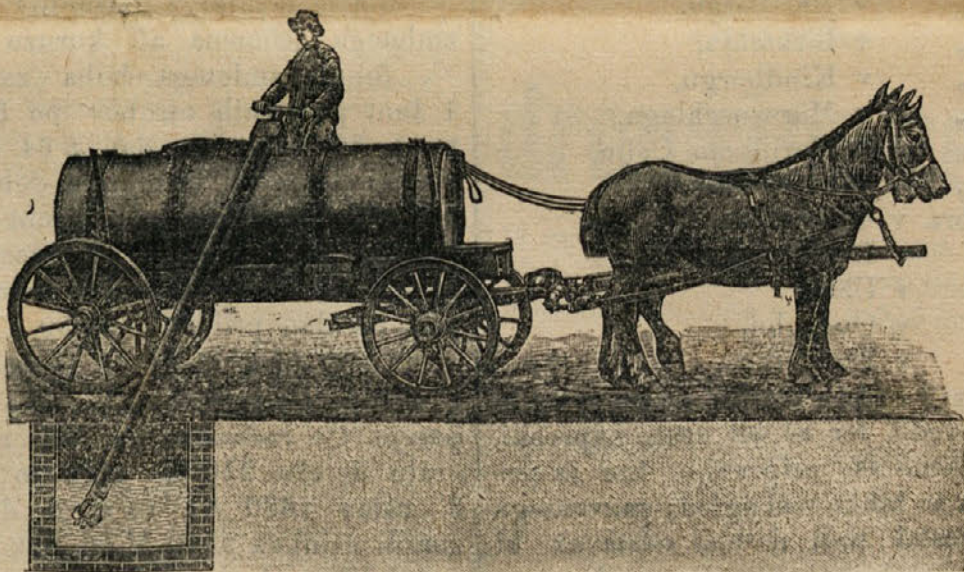
Pod. 1. Navadna sesalka za vodo in gnojnico, ktera je bila na nemški kmetijski družbi v Berolinu spoznana za najboljšo.
