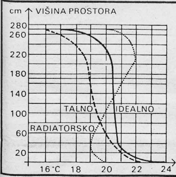
Temperatura prostora po vertikali pri različnem ogrevanju
