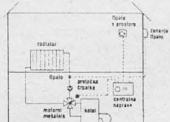
Regulacija temperature z zunanjim tipalom
