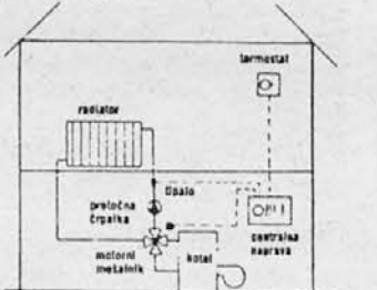
Regulacija temperature v prostoru
