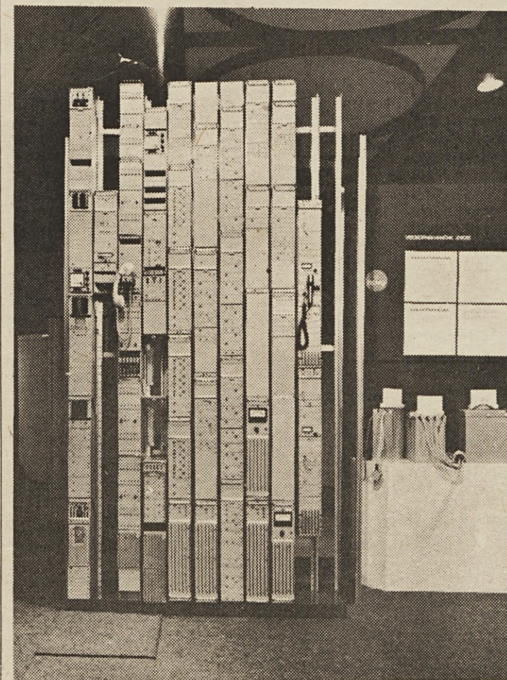
Večkanalni visokofrekvenčni telefonski sistem za prenos podatkov
