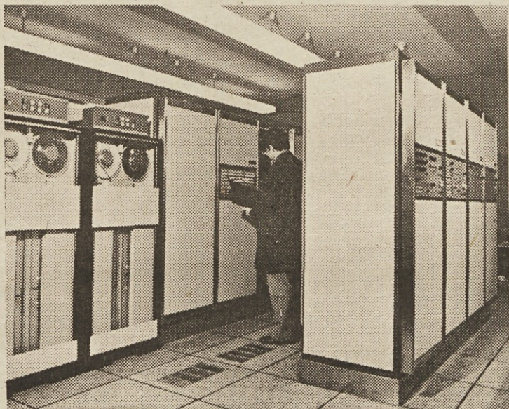
Elektronski računalnik za avtomatsko elektronsko telefonsko centralo Metaconta 10 C telefonske centrale v Ljubljani
