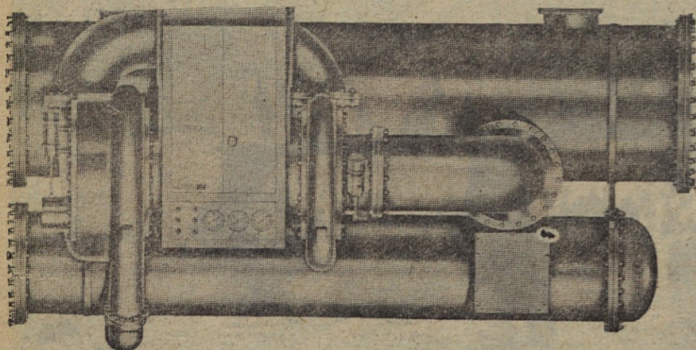
V hladilni centrali bosta v končni fazi instalirana dva hermetična dvostopenjska turbokompresorja s hladilno zmogljivostjo po Q:1.500.000 kcal/h
