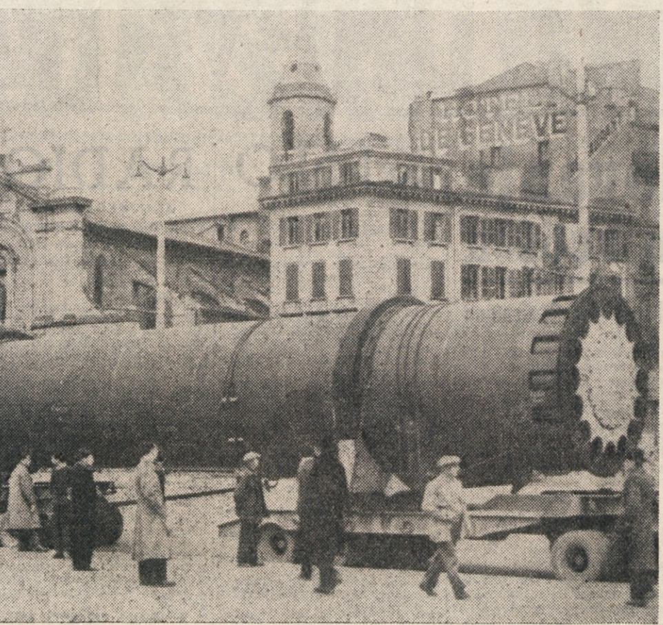
V Marseille so pripeljali velikanski hladilnik "Traylor", ki ga bodo uporabljali v rudniku Pechiney. Hladilnik je 22 m dolg in 75 ton težak. Na sliki vidimo del hladilnika na marsejskih ulicah
